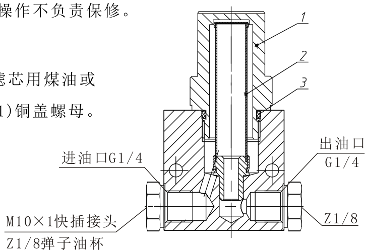
LYQ6型油脂滤油器
